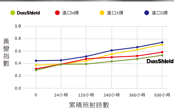
烤漆保護膜抗黃變測試 - 黃變指數變化
